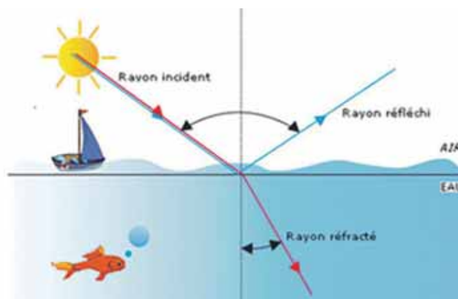
Fig. 1. Source : https://www.maxicours.com/se/cours/refraction-et-reflexion-totale/ . Ce phénomène de réflexion-réfraction existe pour les types d'ondes.
