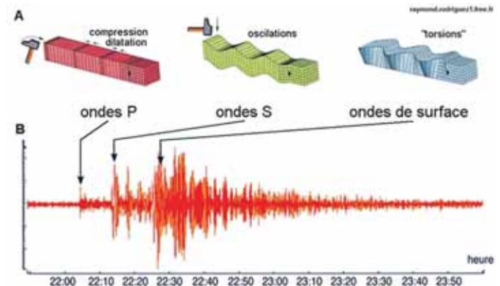
Fig. 2. A. Les trois types d'ondes sismiques. B. Enregistrement d'un sismographe. Source : https://actugeologique.fr/2019/02/les-ondes-sismiques/
