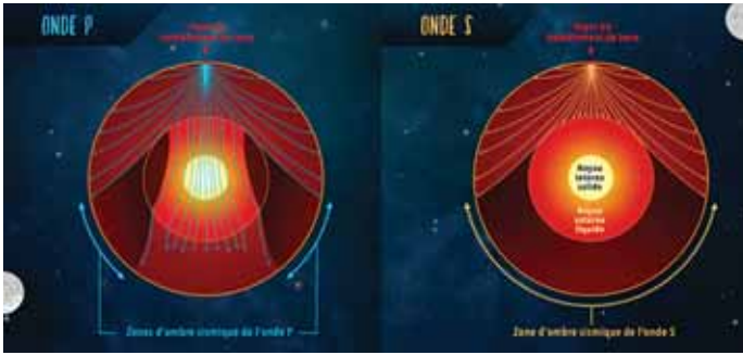
Figure 3. Ondes P et S se propageant à travers la Terre et permettant de déterminer la structure interne de la Terre. (© Arteclic). http://marsatschool.ethz.ch/fr/mision/7/index.html
